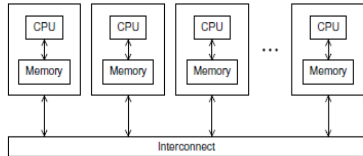
Memoria distribuita
